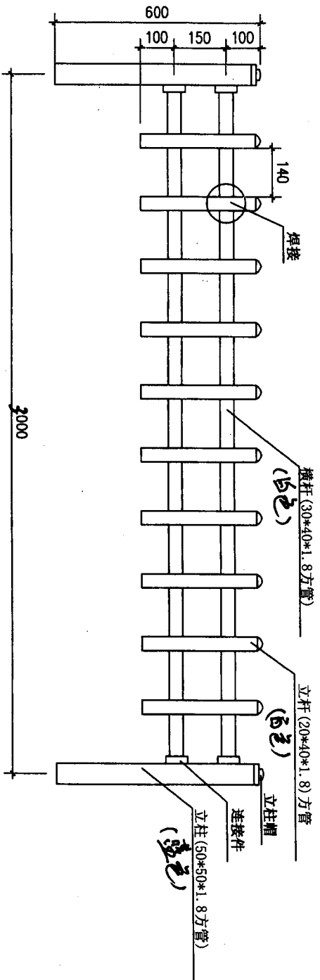
护栏三 立面图 (单位: mm)
