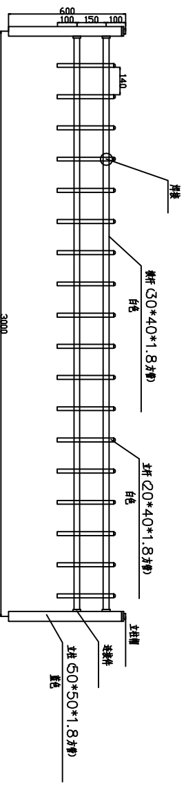
防护栏一 立面图 (单位:mm)
